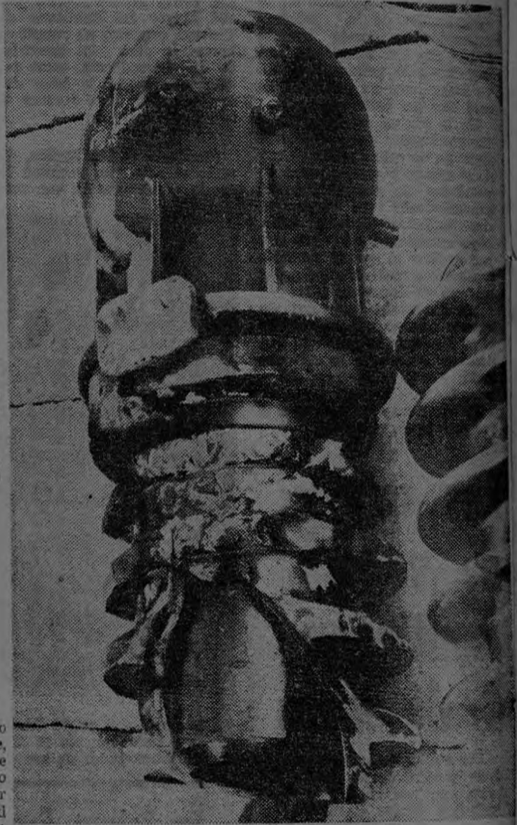
INTERRUPTOR QUE EXPLOTO. — La gráfica recoge al interruptor que explotó ayer a las seis de la tarde en la Subestación de Colima y que provocó un apagón en la capital por cerca de una hora. Esto causó además daños a dos pararrayos de la Planta de Cachí. El interruptor fue reparado anoche mismo.
